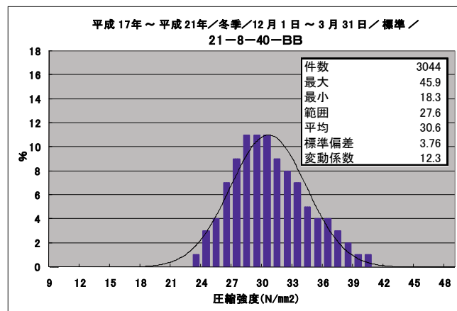
図1-4 圧縮強度ヒストグラムH17~H21(冬季)
