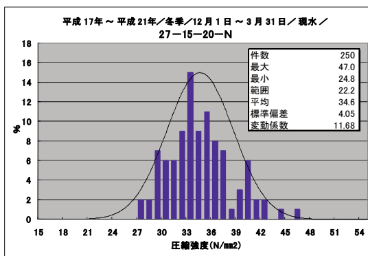
図2-3 圧縮強度ヒストグラム H17~H21 (冬季) 現場水中養生
