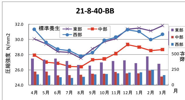
図1-2 圧縮強度の月別推移(地区別)H17~H21
