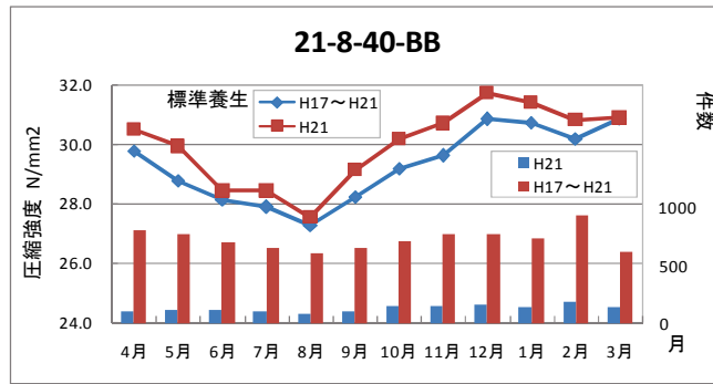
図1-1 圧縮強度の月別推移(全県)H17~H21
