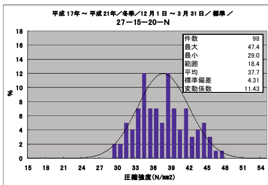
図2-5 圧縮強度ヒストグラム H17~H21 (冬季) 標準養生
