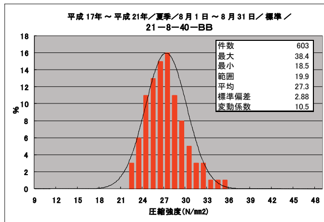
図1-3 圧縮強度ヒストグラムH17~H21(夏季)
