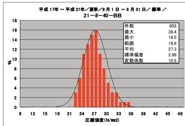
図1-3 圧縮強度ヒストグラムH17~H21(夏季)
