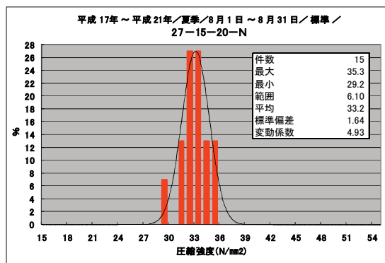
図2-4 圧縮強度ヒストグラム H17~H21 (夏季) 標準養生
