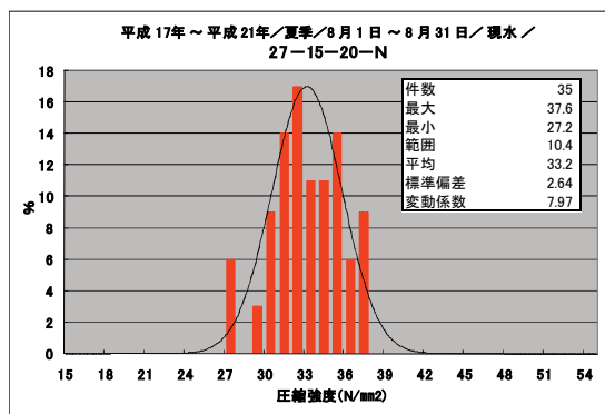
図2-2 圧縮強度ヒストグラム H17~H21 (夏季) 現場水中養生
