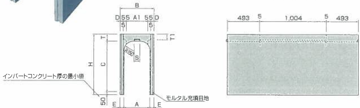
側面図
