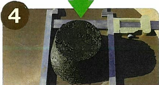
攪拌後 フロー試験 (100mm、運搬可)
