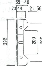
正面図
