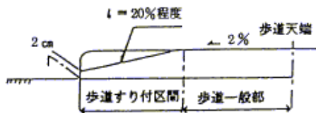
a-a' 断面図
