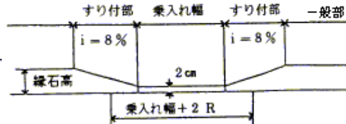
b-b' 正面図
