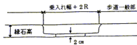
b-b' 正面図
