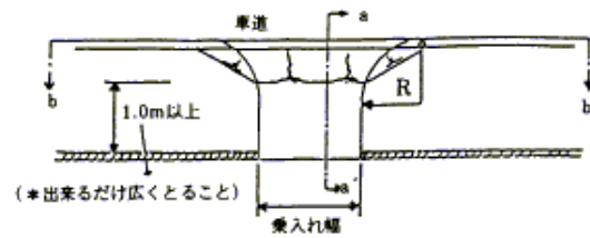
平面図
